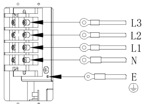
Рисунок 12 Підключення до трифазної електромережі
